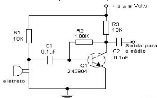
Pré para amplificação de excelente ganho.
