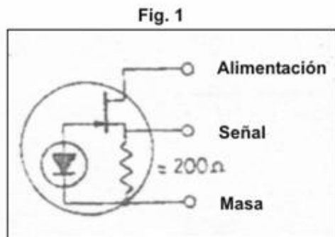
Cicuito de micrófono electreto
