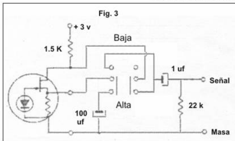
Modificación para aumentar la tensión de salida. La tensión debe de estar apropiadamente desacoplada.
