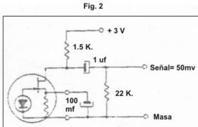
Modificación para aumentar la tensión de salida. La tensión debe de estar apropiadamente desacoplada.
